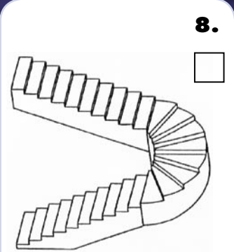
Treppe 1x 180° gewendelt ohne Podest
